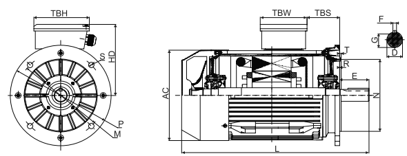
IM B5 - D Flange
